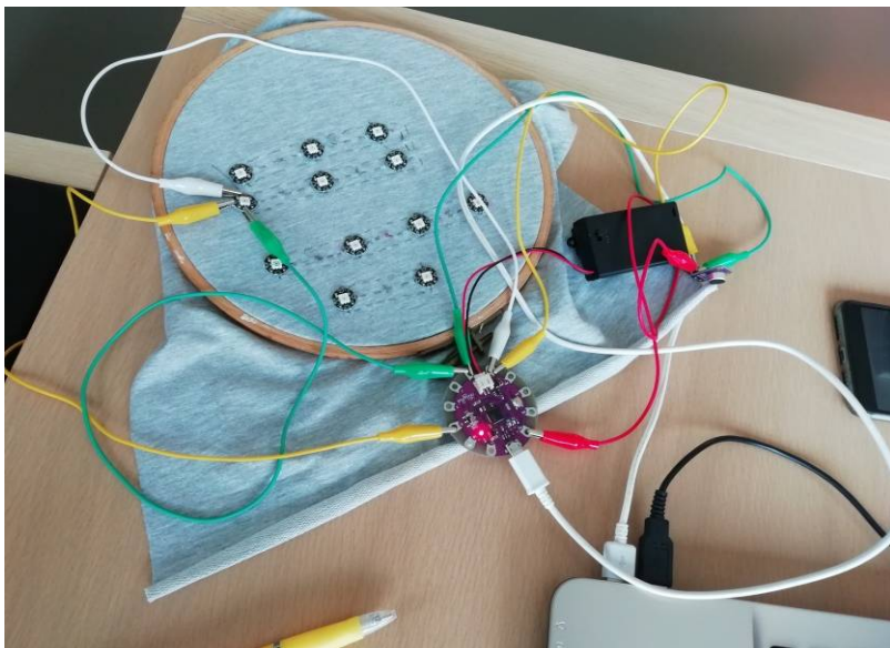
Pokus č. 6. - Strojové vyšívání a ruční přišíť LED diod , kontrolní práce
